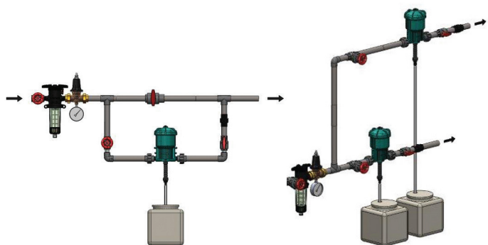
Instalação bypass
