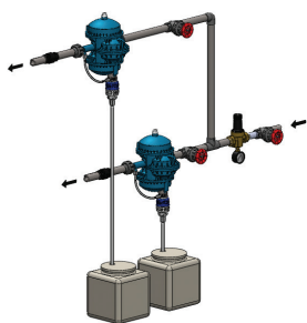
Instalação dupla fixa inline
