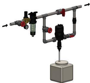
Instalação bypass
