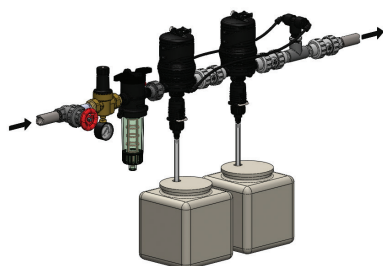
Instalação dupla fixa inline
